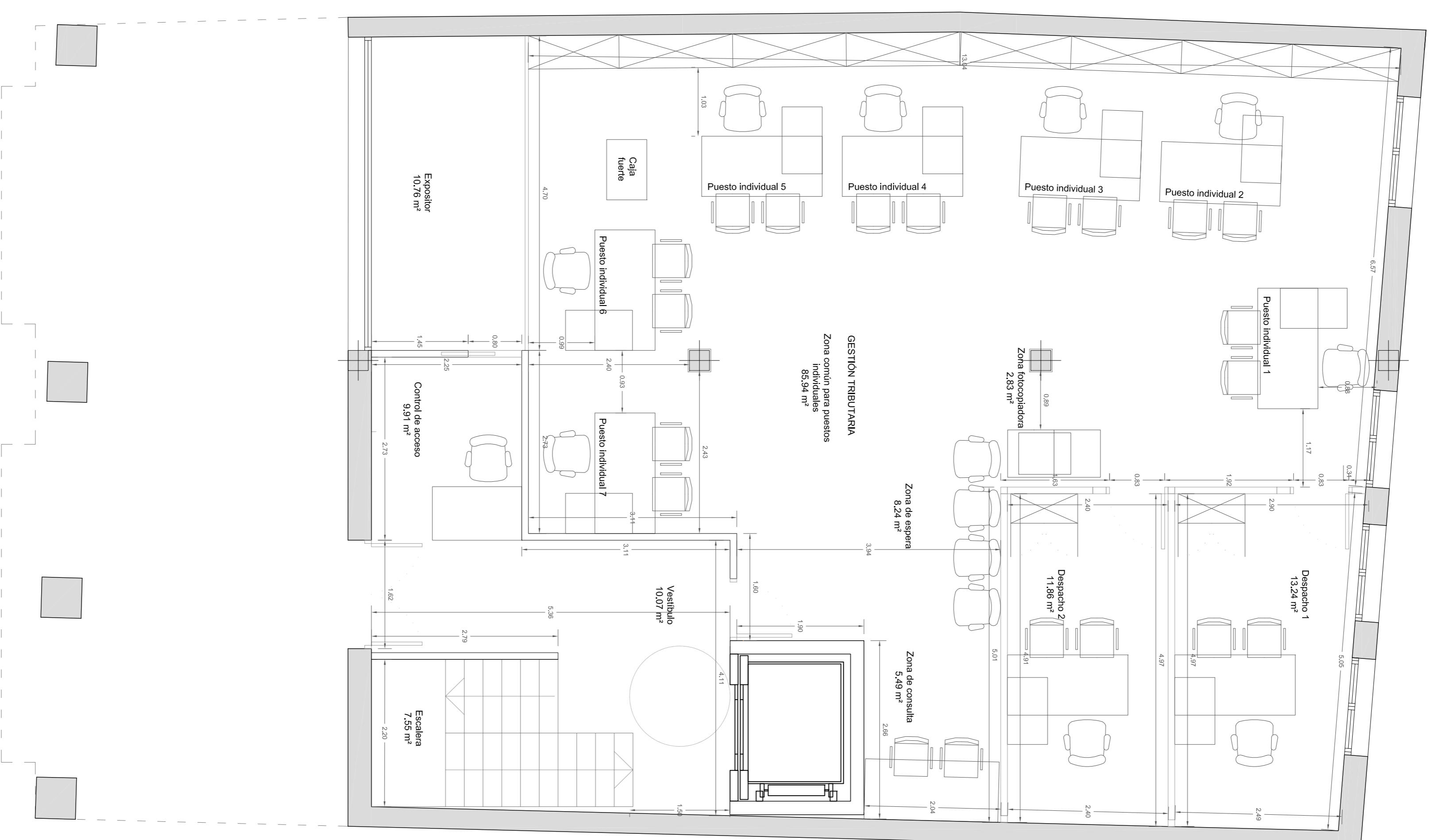
PLANTA BAJA
