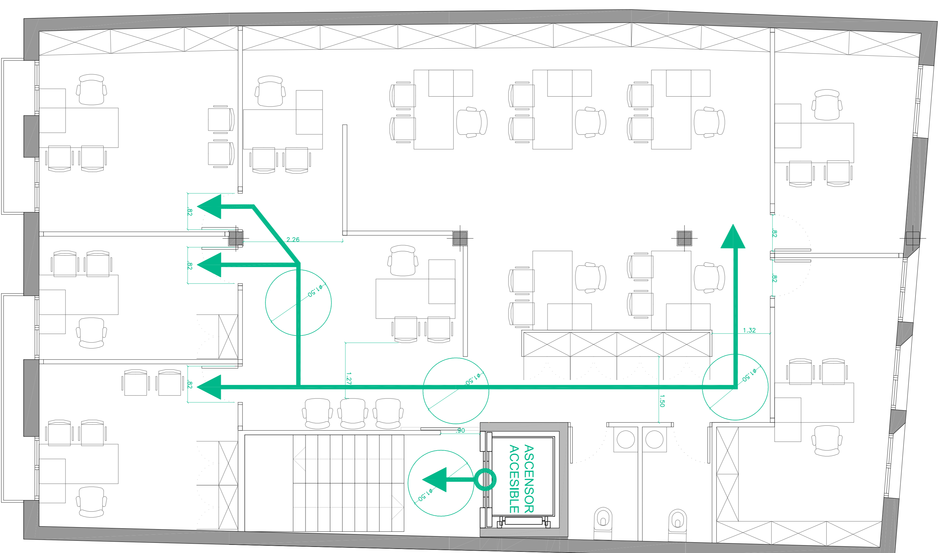
PLANTA SEGUNDA
