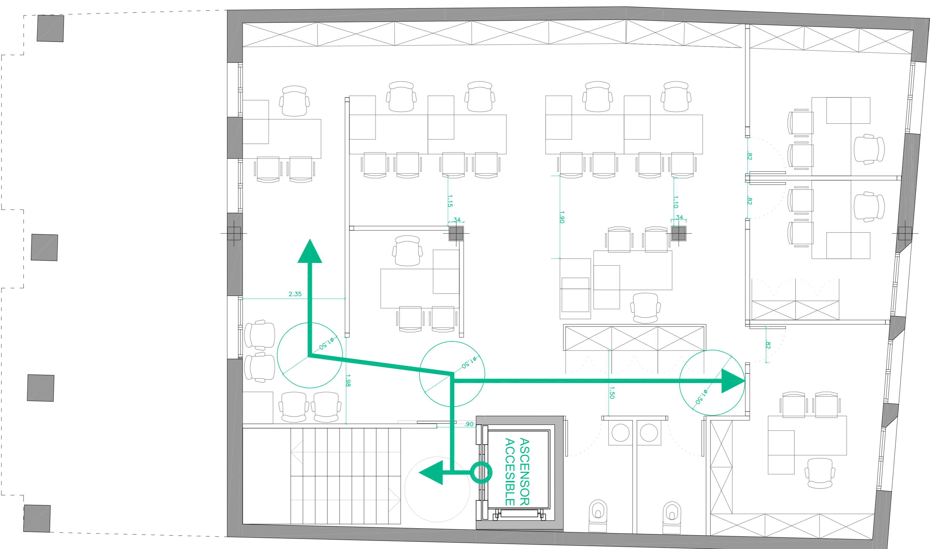
PLANTA PRIMERA
